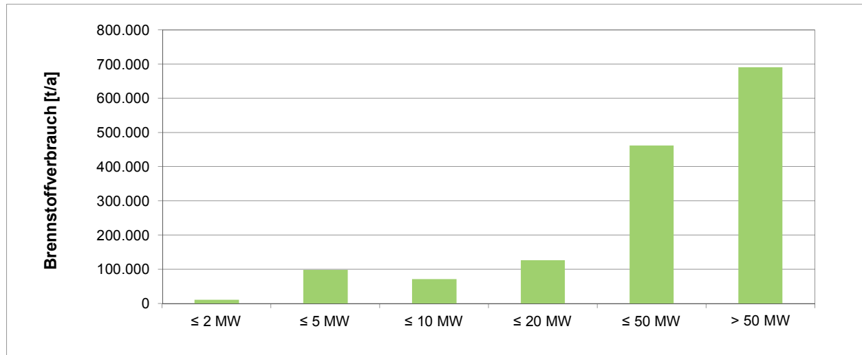
Abb. 11: Brennstoffverbrauch der Holzfeuerungsanlagen > 1 MW nach Größenklassen
