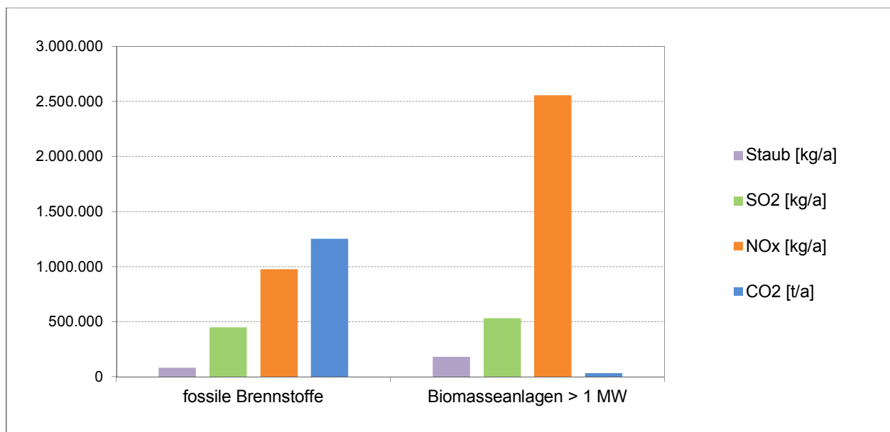
Abb. 15: Emissionsvergleich zwischen Holzfeuerungen oberhalb 1 MW und fossil befeuerten Anlagen
