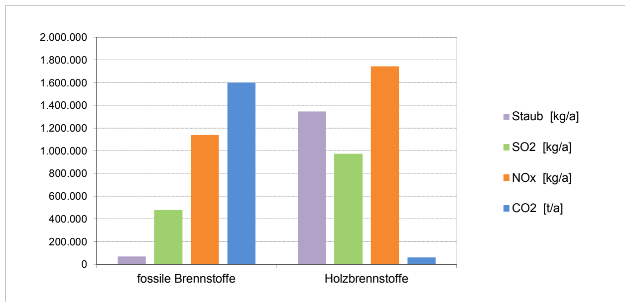
Abb. 14: Emissionsvergleich zwischen holz- und fossil befeuerten Heizanlagen < 1 MW
